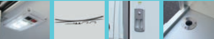
■庫内灯&非常ブザー ■強化リヤスプリング (三菱純正4枚リフ) ■引戸式サイドドア ロックレバー ■水抜き穴 (左前)
